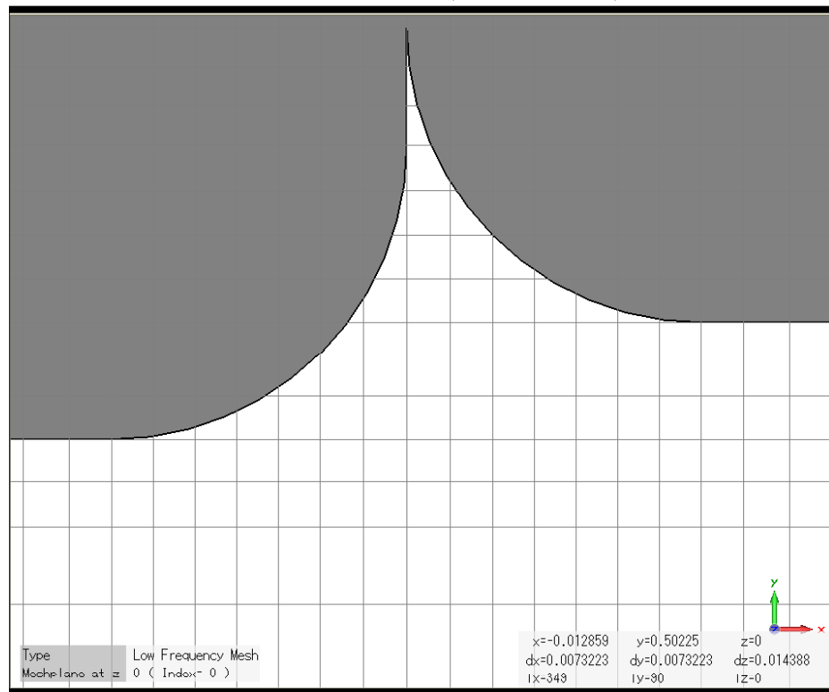
RAPL=2(default)
