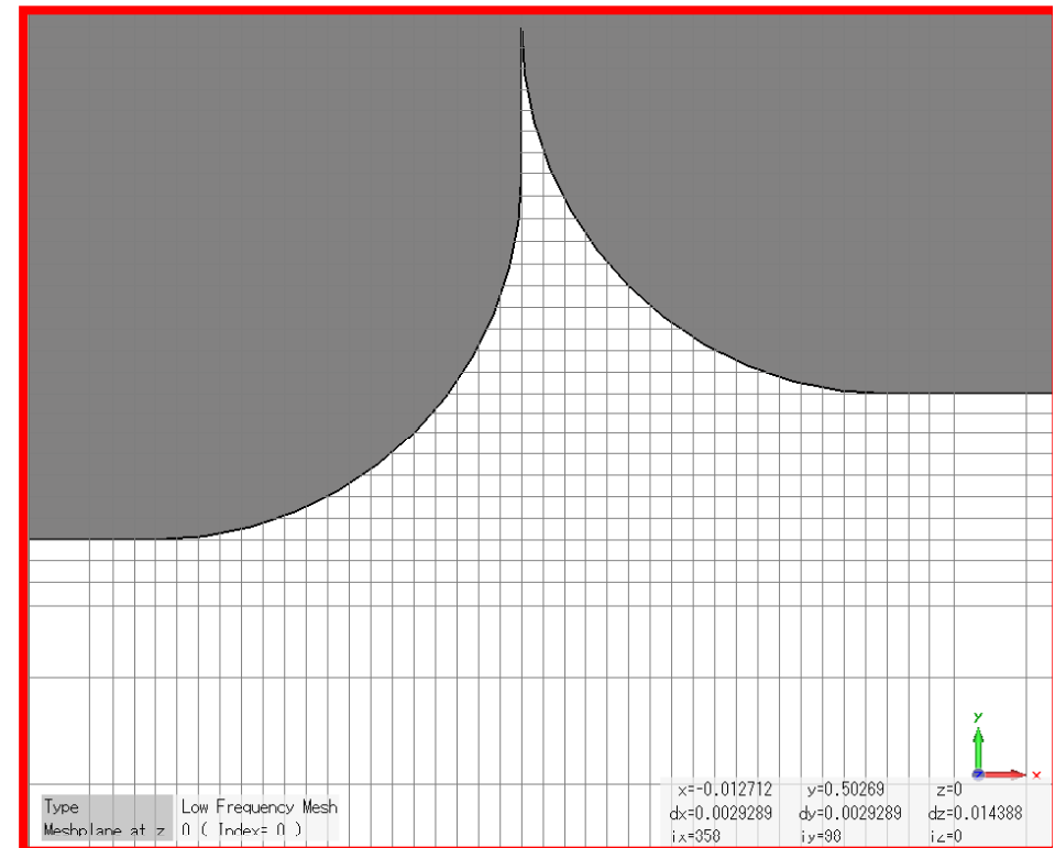
RAPL=5
