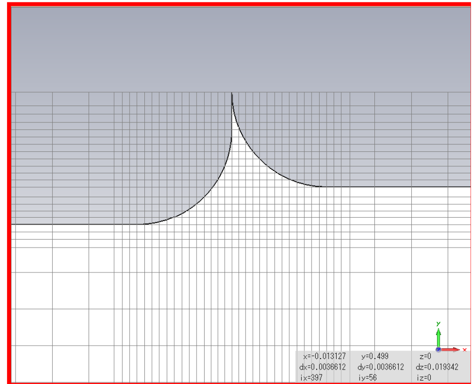
RAPL=5
